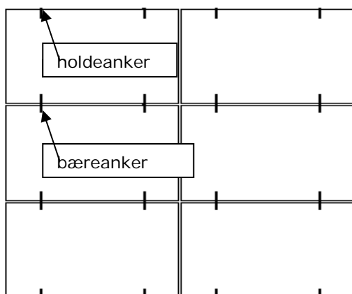
Bære og holdeankre i horizontale fuger
