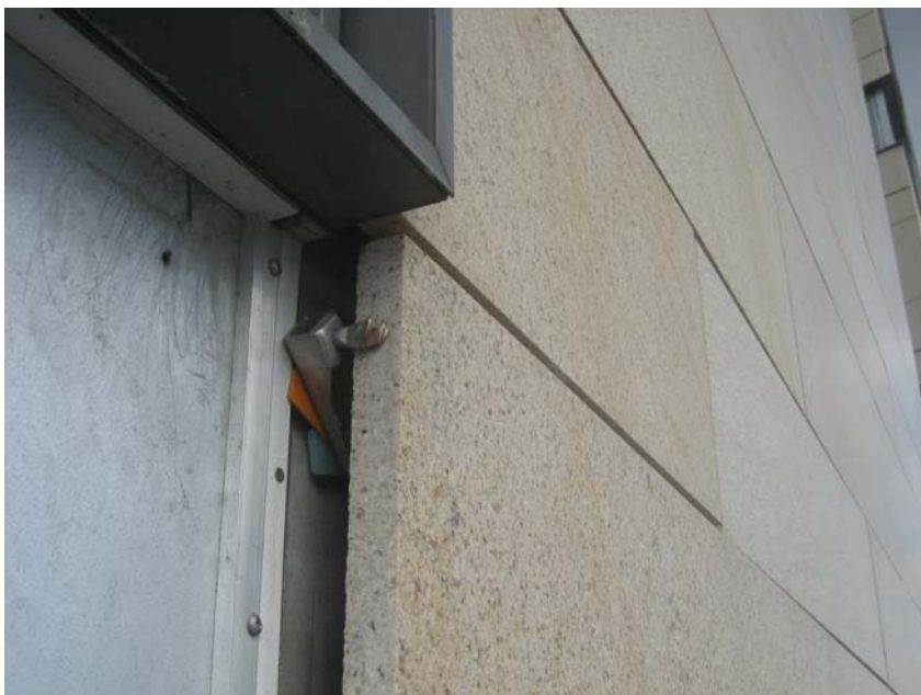
Foto. 4, 30 mm granitplader opsat med dorn på et holdeanker i vertikalfuge.
